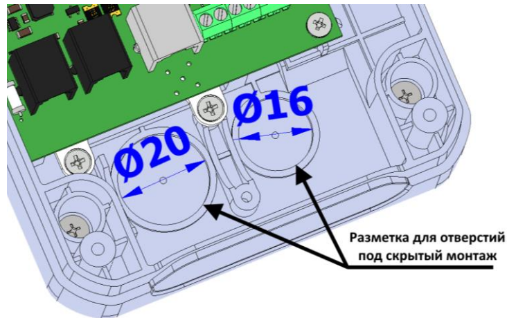
Рисунок 4 – Разметка под отверстия для скрытого монтажа
