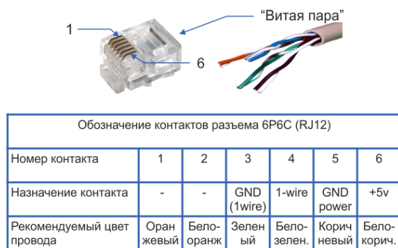
Рисунок 4 – Обозначение разъемов 6P6C (RJ12)
