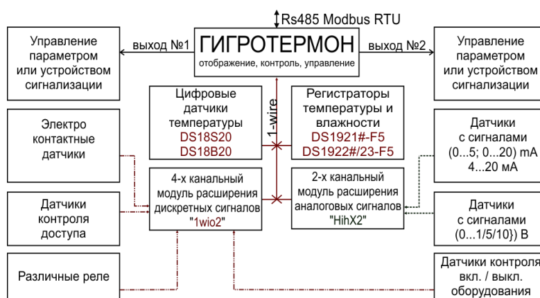
Рисунок 3 – Схема подключения устройств к прибору
